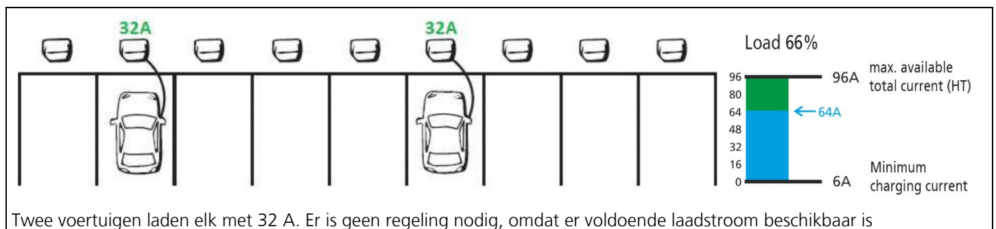
Afb. 10: Voorbeeld lastmangement bedrijfstoestand 1
