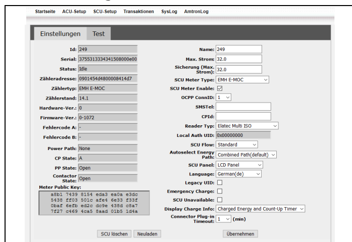
Abb. 5: SCU-Setup – Einstellungen
