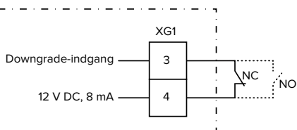
Fig. 13: Principskema: Tilslutning af en ekstern omskifterkontakt (standardindstilling: NO)
