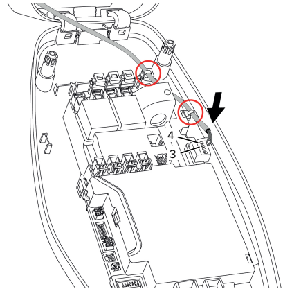
Εικ. 12: Σύνδεση εισόδου περιορισμού ισχύος
