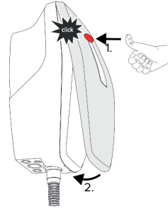
Εικ. 18: Τοποθέτηση του μπροστινού καλύμματος - 1
