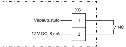
Kuva 15: PeriaatekytKentäkaavio: vapautustulo
