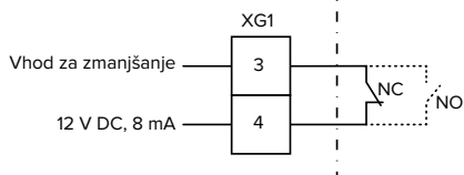
sl. 13: Osnovna vezalna shema: Priključitev zunanega preklopnega kontakta (standardna nastavitev: NO)
