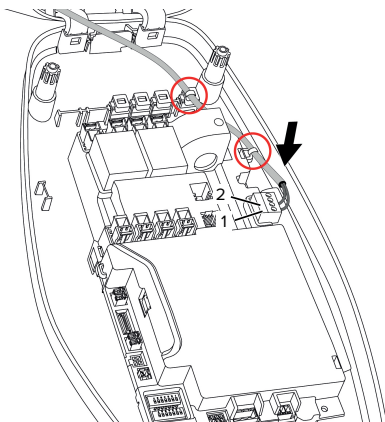
sl. 14: Priključek vhoda za sprostitvev
