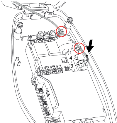
Abb. 12: Anschluss Downgrade-Eingang
