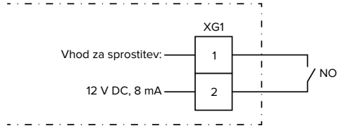
sl. 15: Osnovna vezalna shema: Vhod za sprostitvev
