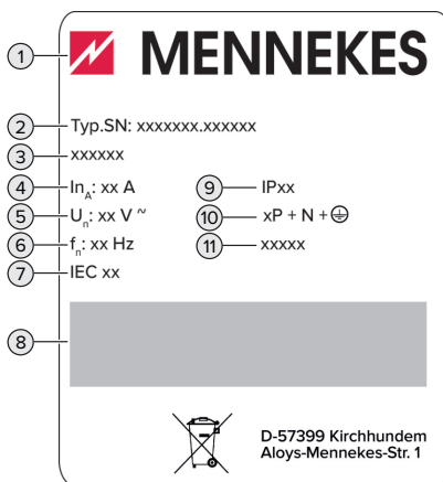
Afb. 1: Producttypeplaatje (voorbeeld)
