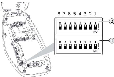
Afb. 11: Dipschakelaar (uitleveringstoestand)
