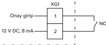
Şek. 15: Prensipsel devre şeması: Onay girişi
