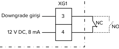
Şek. 13: Prensiptel devre şeması: Harici bir şalter kontaklarının bağlanması (standart ayar: NO)
