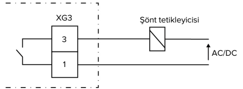
Şek. 10: Prensiyel devre şeması: Harici bir şönt tetikleyicisinin bağlanması
