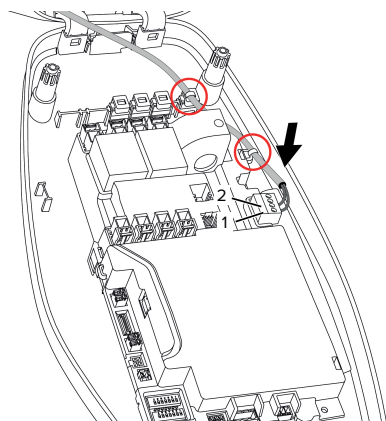
Fig. 14: Conexión entrada de habilitación
