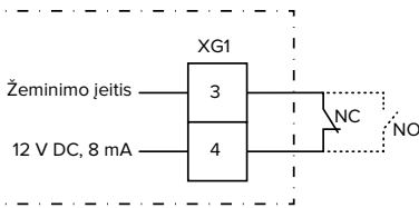
Pav. 13: Principinė sujungimo schema: išorinio jungimo kontakto jungties prijungimas (standartinis nustatymas: NO)
