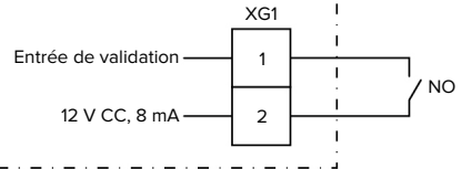
Fig. 15 : Schéma de principe : Entrée de validation
