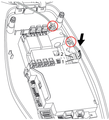
Abb. 14: Anschluss Freigabe-Eingang
