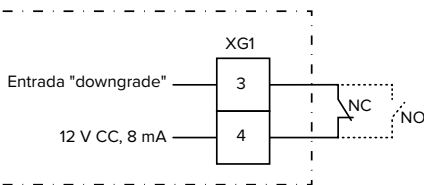
Fig. 13: Esquema de princípio: ligação de um contacto de comutação externo (configuração padrão: NO)
