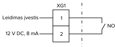
Pav. 15: Principinė sujungimo schema: leidimo jėgimas
