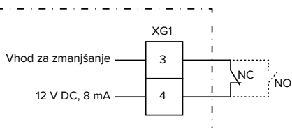
sl. 13: Osnovna vezalna shema: Priključitev zunanjega preklopnega kontakta (standardna nastavev: NO)
