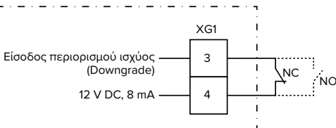
Εικ. 13: Διάγραμμα συνδεσμολογίας: Σύνδεση εξωτερικής επαφής μεταγωγής (βασική ρύθμιση: NO)
