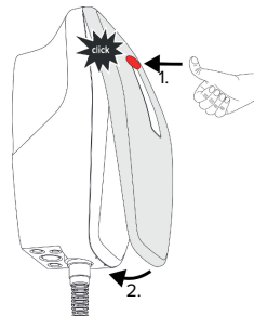
Fig. 18 : Monter le cache frontal - 1
