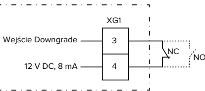
Ilustr. 13: Schemat blokowy: podłączenie zewnętrznego styku przełączającego (ustawienie standardowe: NO)
