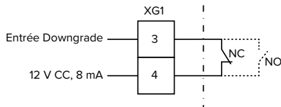
Fig. 13 : Schéma de principe : raccordement d'un contact électrique externe (réglage par défaut : NO)
