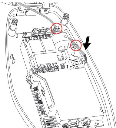
Fig. 14: Tilkobning frigivelsesindgang
