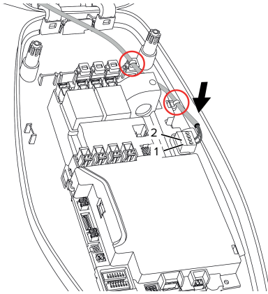
Şek. 14: Onay girişi bağlantısı
