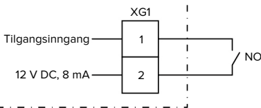
Fig. 15: Prinsipielt koblingsskjema: Tilgangsinngang
