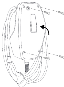
Fig. 16: Stenge produktet
