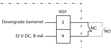
13. Ábra: Elvi kapcsolási rajz: Külső kapcsolóérintkező csatlakoztatása (normál beállítás: NO)
