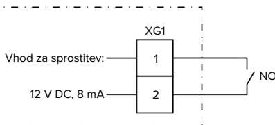
sl. 15: Osnovna vezalna shema: Vhod za sprostitve
