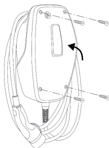
Pav. 16: Uždaryti gaminį
