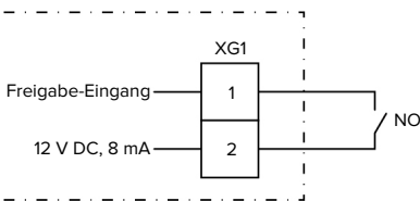
Abb. 15: Prinzipschaltbild: Freigabe-Eingang
