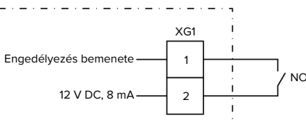
15. Ábra: Elvi kapcsolási rajz: Engedélyezés bemenete
