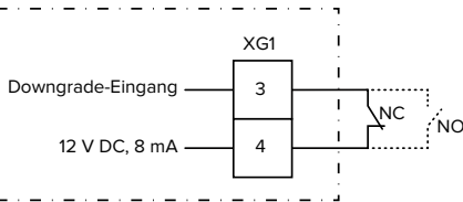
Abb. 13: Prinzipschaltbild: Anschluss eines externen Schaltkontakts (Standard-Einstellung: NO)
