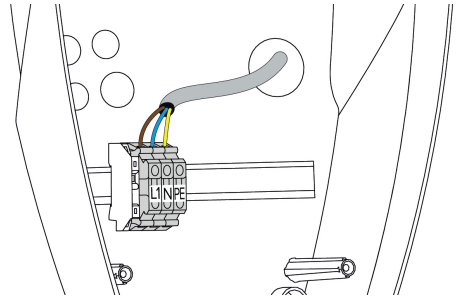
Kuva 8: Jännitesyötön liitäntä
