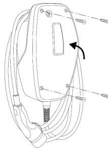
Kuva 16: Tuotteen sulkeminen
