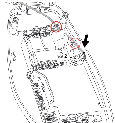
Fig. 14 : Raccordement de l'entrée de validation
