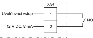
Obr. 15: Základní schéma zapojení: uvolňovací vstup
