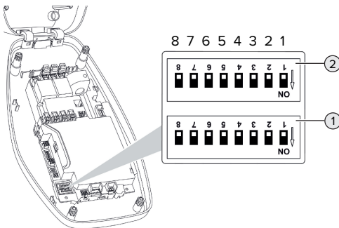
Fig. 11: DIP-brytare (leveranstillstånd)
