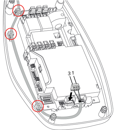
Şek. 9: Şönt tetikleyicisi bağlantısı
