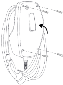
Abb. 16: Produkt schließen
