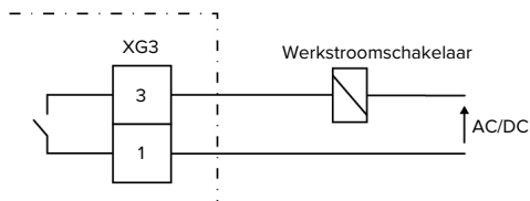
Afb. 10: Principe-schakelschema: Aansluiting van een externe werkstroomsschakelaar
