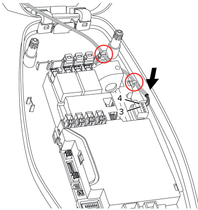
Fig. 12: Conexión entrada Downgrade
