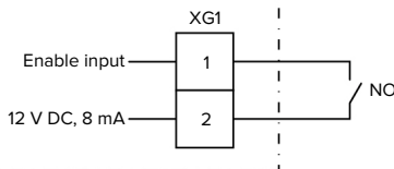
Fig. 15: Schematic circuit diagram: Enable input
