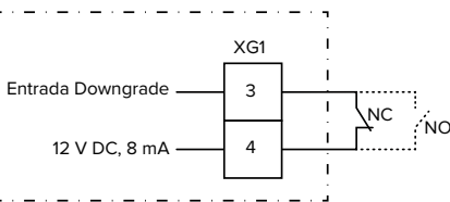
Fig. 13: Esquema de principio: Conexión de un contacto de conmutación externo (ajuste estándar: NO)
