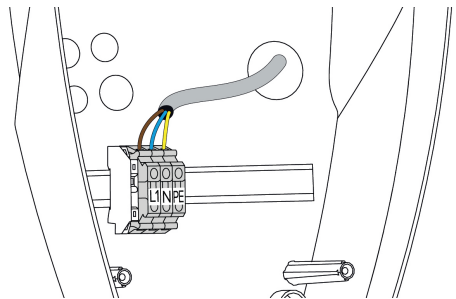
Afb. 8: Aansluiting stroomvoorziening
