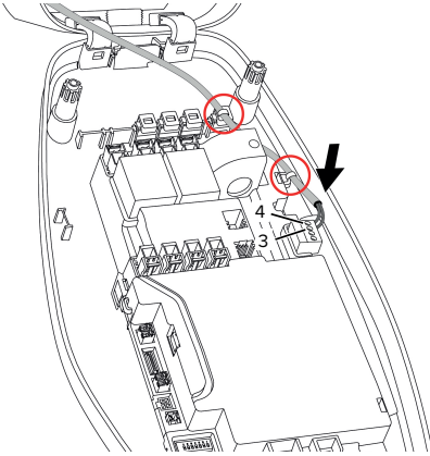
Kuva 12: Downgrade-tulon liittäminen
