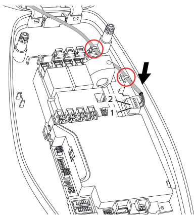
Obr. 14: Připojení uvolňovacího vstupu
