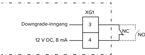
Fig. 13: Prinsipielt koblingsskjema: tilkobling av en ekstern bryterkontakt (standardinnstilling: NO)
