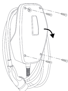
Kuva 5: Tuotteen avaaminen
