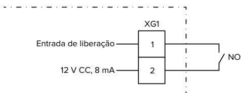
Fig. 15: Esquema de princípio: Entrada de liberação
