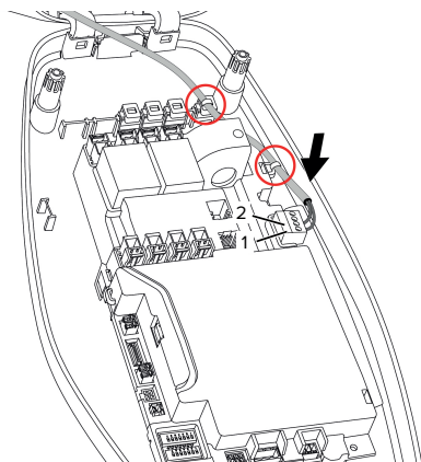
Fig. 14: Anslutning av aktiveringsingång
