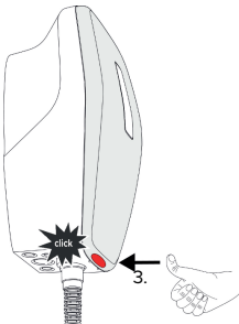
Kuva 19: Front Coverin kiinnitys – 2
