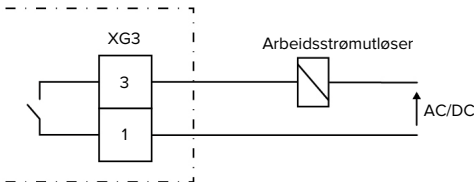
Fig. 10: Prinsipielt koblingsskjema: Tilkobling av en ekstern arbeidsstrømutløser
