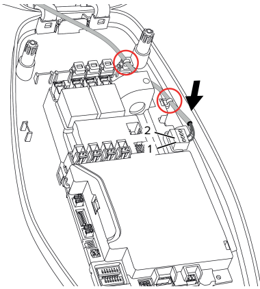
Kuva 14: Liitäntä vapautustulo
