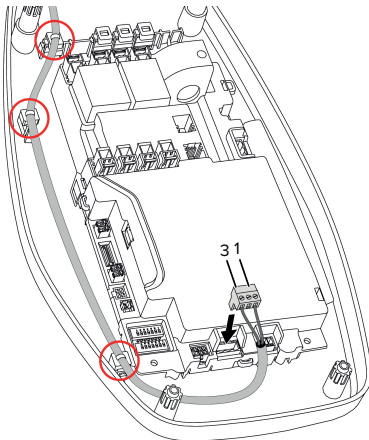
Afb. 9: Aansluiting arbeidsstroomactiveringsschakelaar
