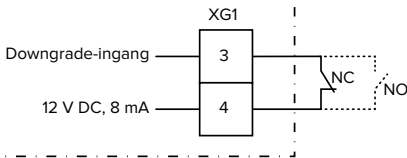
Afb. 13: Principe-schakelschema: Aansluiting van een extern schakelcontact (standaardinstelling: NO)
