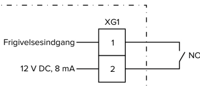
Fig. 15: Principskema: Frigivelsesindgang
