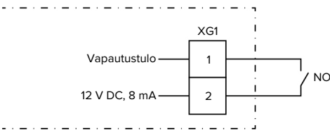
Kuva 15: Periaatekytkentäkaavio: vapautustulo
