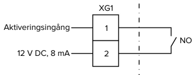
Fig. 15: Principkopplingsschema: Aktiveringsingång
