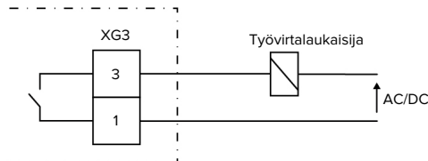
Kuva 10: Periaatekytkentäkaavio: ulkoisen työvirran laukaisijan liitännät
