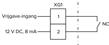
Afb. 15: Principe-schakelschema: Vrijgave-ingang
