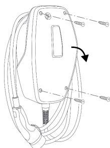
Fig. 5: Åpne produktet
