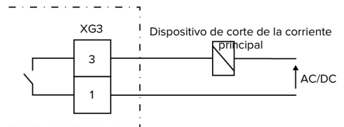
Fig. 10: Esquema de principio: Conexión de un dispositivo de corte de la corriente principal externo
