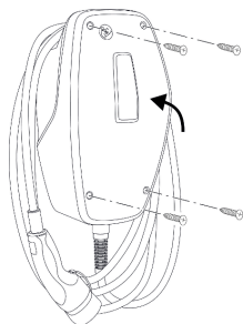
Fig. 16: Cierre del producto
