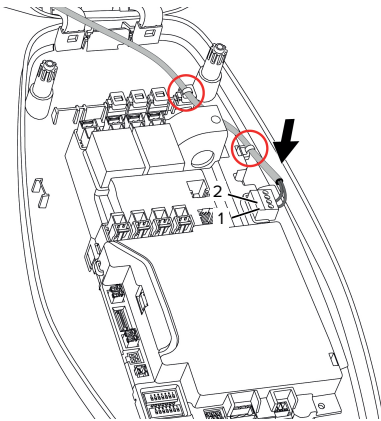
Afb. 14: Aansluiting vrijgave-ingang
