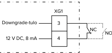
Kuva 13: Periaatekytkentäkaavio: ulkoisen kytkentäkontaktin liittäminen (vakioasetus: NO)
