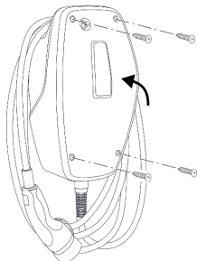
Fig. 16 : Fermeture du produit
