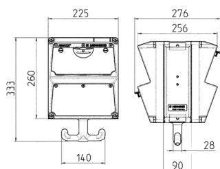
Schéma 1 MB 630
