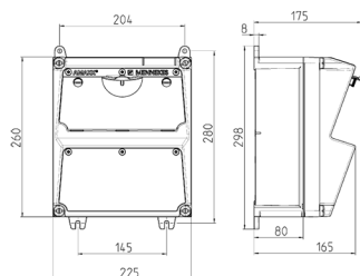
Schéma 1 MB 521
