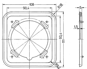
Schéma 1 MB 363 Dim. en mm
